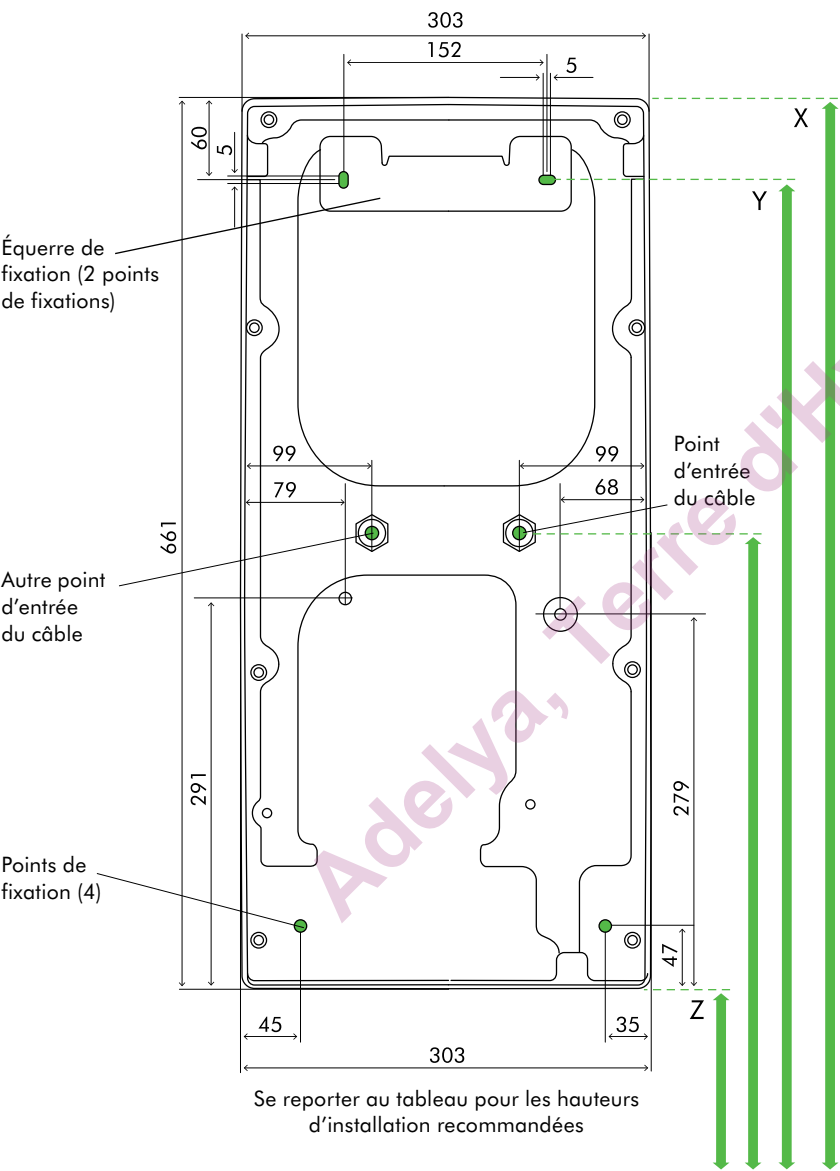
SCHÉMA DU DOS DE L'APPAREIL
